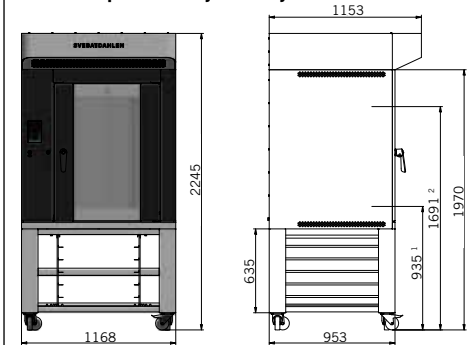
Boceto dimensional del SR240 con carro para bandejas debajo.
